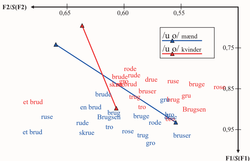
Figur 3: Middelværdier af normaliserede formanter, hhv. F1 (tungsænkning) og F2 (fremskydning), for udtalen af forskellige ords u-/o-vokaler.
