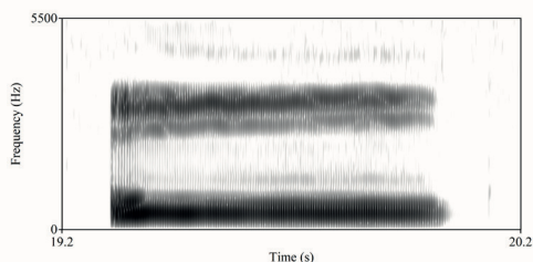
Figur 2: Spektrogram af samme talers [o].
