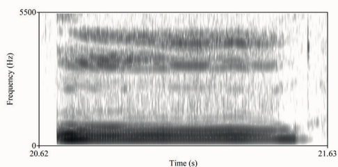
Figur 1: Spektrogram af en talers [u].
